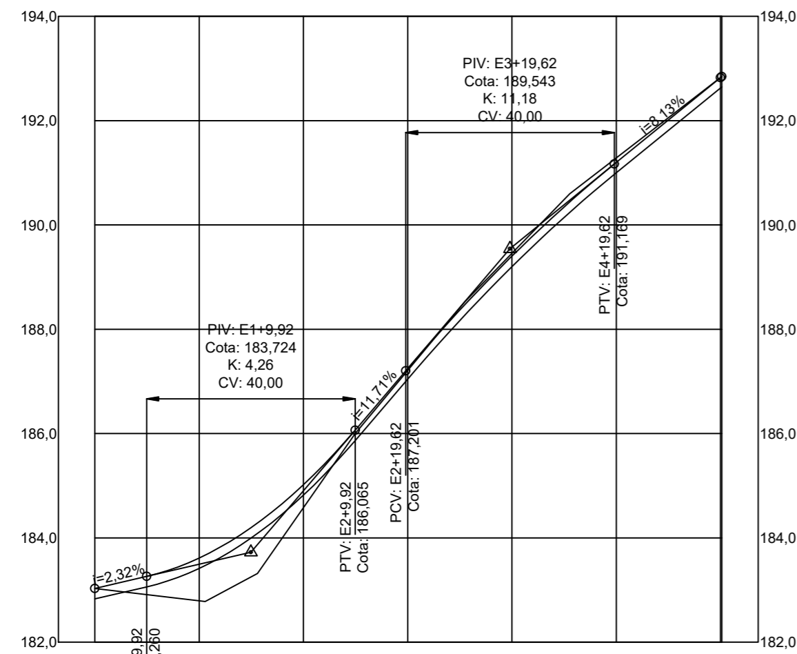
RUA PROJETADA 01 - E0+0 ATÉ E6+0,24 PERFIL LONGITUDINAL - ESC.: V=1:100 H=1:1000
