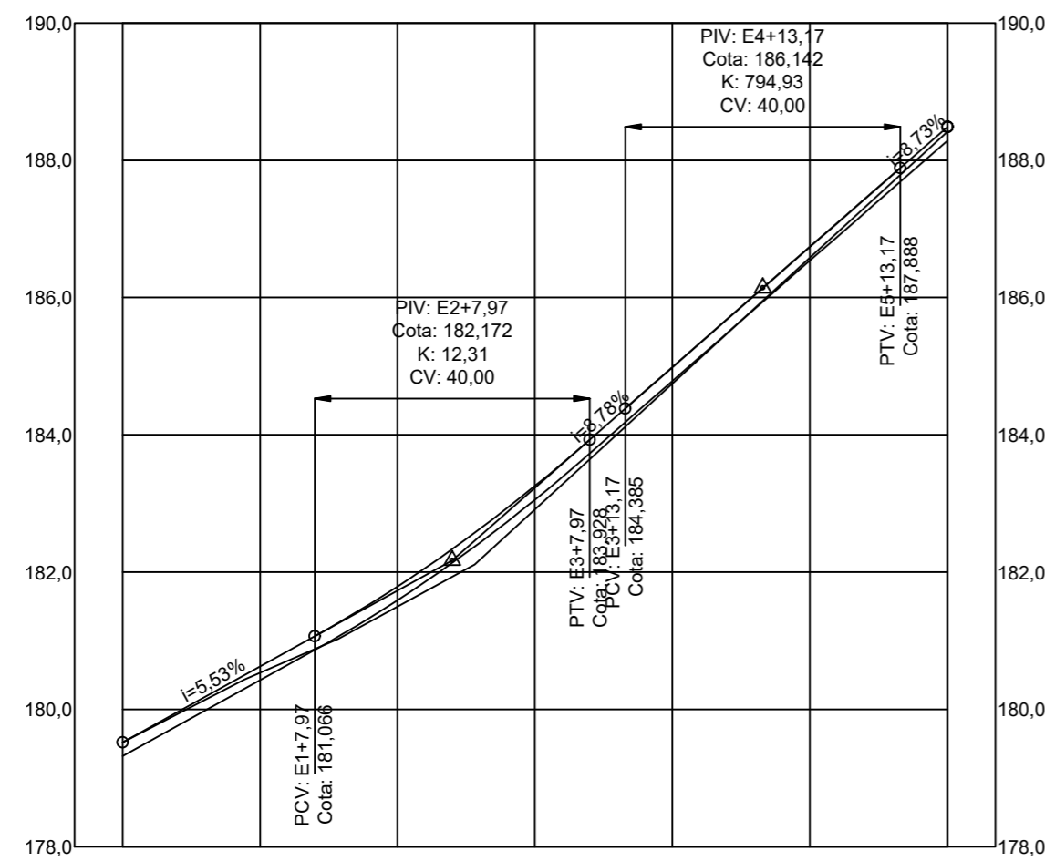
RUA PROJETADA 02 - E0+0 ATÉ E6+0,03 PERFIL LONGITUDINAL - ESC.: V=1:100 H=1:1000
